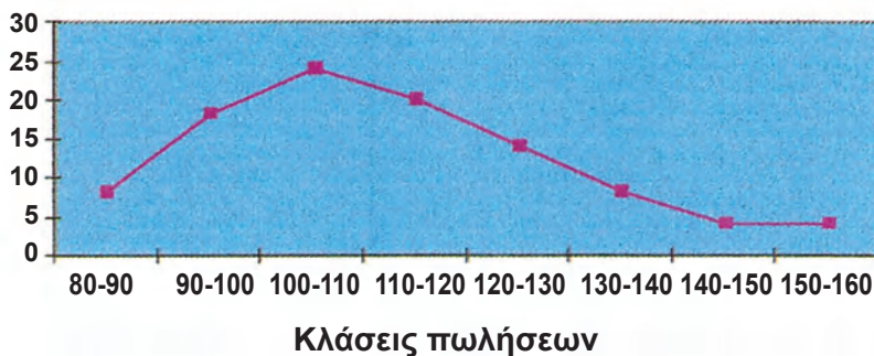
(Σχ. 3.10) Πολύγωνο σχετικών συχνοτήτων.
