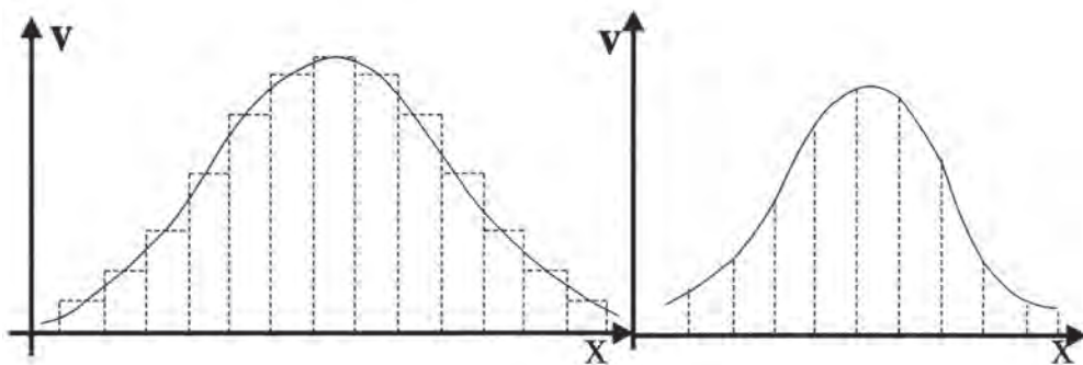
(Σχ. 3.12) Πολύγωνο συχνοτήτων συνεχούς μεταβλητής.
