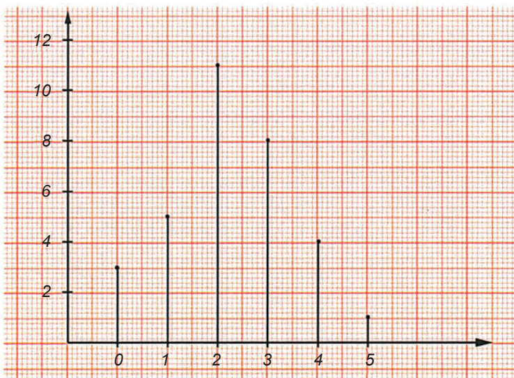
(Σχ. 3.5) Διάγραμμα Συχνοτήτων
