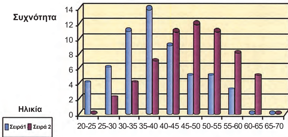
(Σχ. 3.13) Συγκριτικό διάγραμμα συχνοτήτων με κυλίνδρους.
