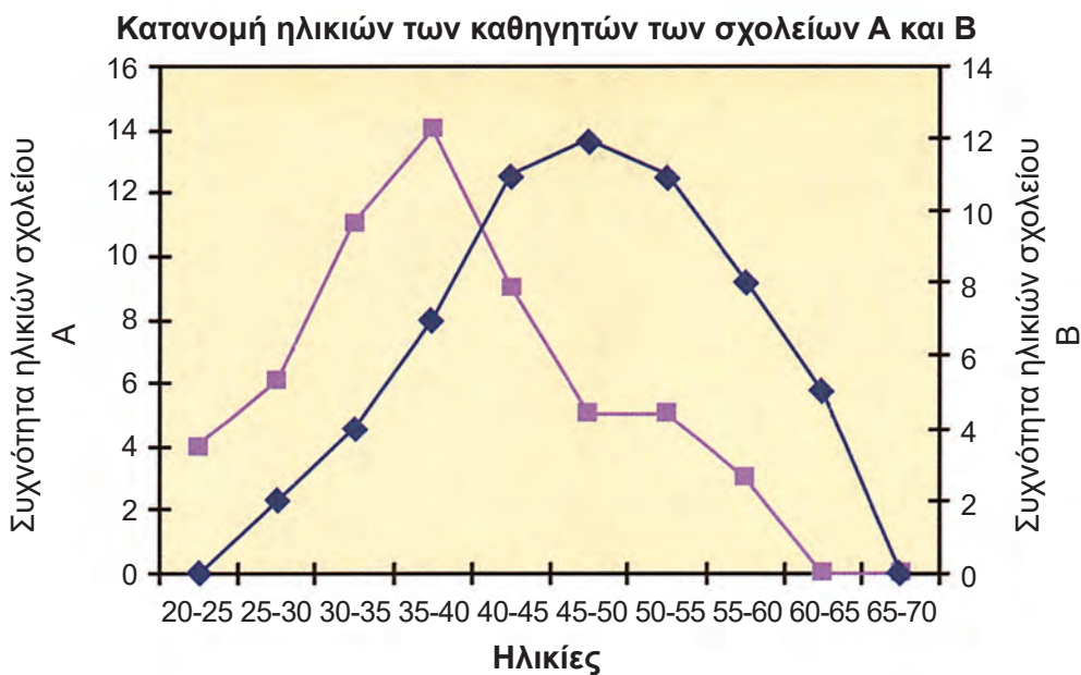
(Σχ. 3.15) Συγκριτικά πολύγωνα συχνοτήτων.
