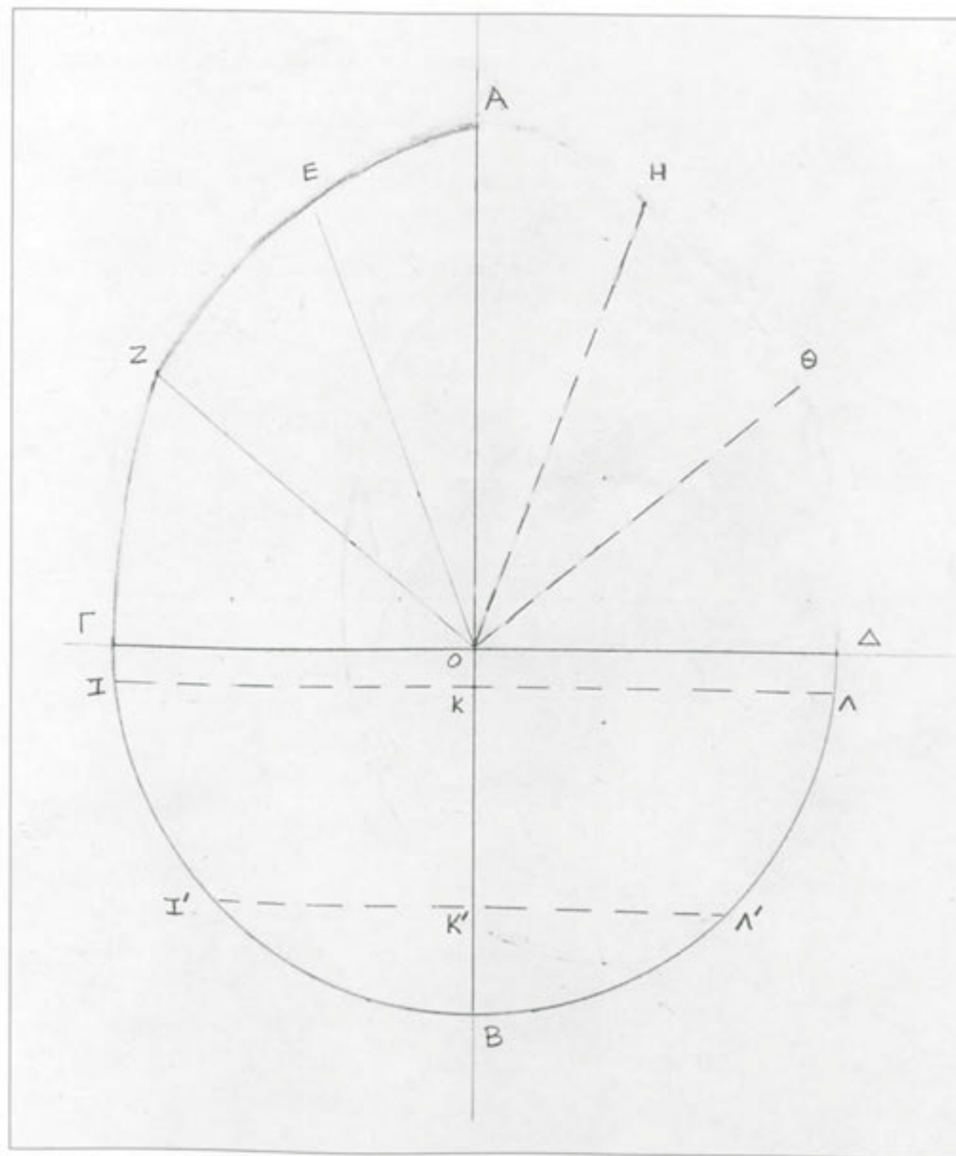
Εικ. 1.77 Γεωμετρική κατασκευή για ειδικό τύπο ωσσιδούς περιδέραιον, σε φυσικό μέγεθος.
